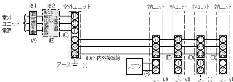
—同時トリプル・フォーシステムの配線—
