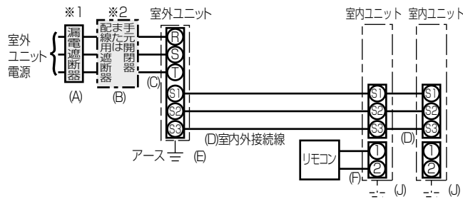
—同時トリプル・フォーシステムの配線—
