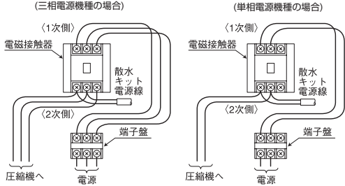
図1: 室外ユニット制御部内 (三相電源機種の場合)
