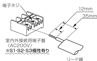
【図32】 〈接続詳細〉
