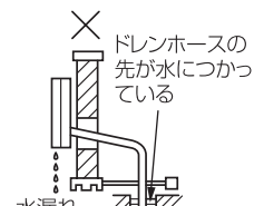
【図21】 排水こう
