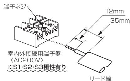
【図32】 〈接続詳細〉
