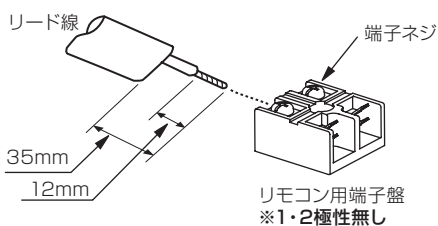
【図31】 〈接続詳細〉
