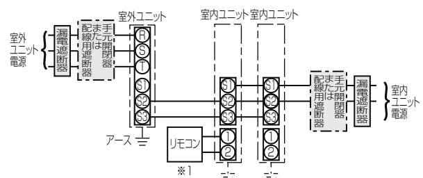
室内ユニットの電源をS1およびS2に接続
