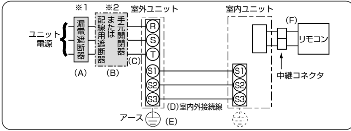
ユニット電源配線
