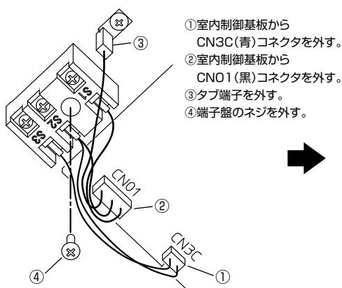
〈室内ユニット端子盤の付け換え〉 (PL-ZRP-EA3, PL-ERP-EA3の場合)
