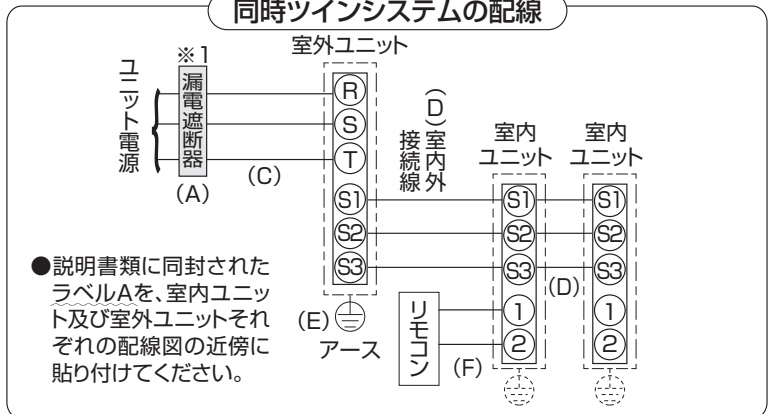
同時ツインシステムの配線
