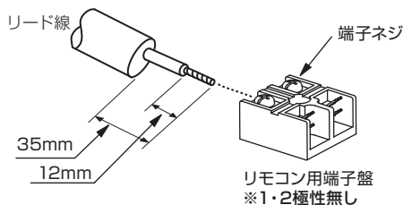
[図31] <接続詳細>
