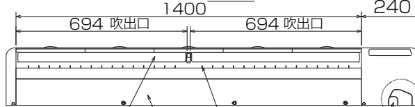
下面図
