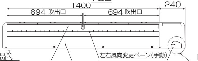
下面パネル (左配管作業時取外し可)
