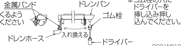
ドレンホース 入れ換える
