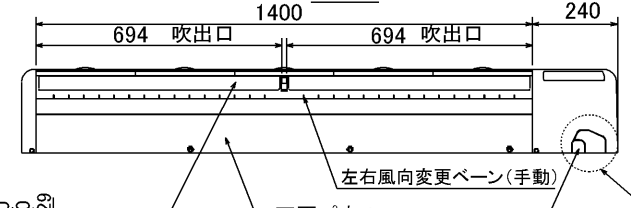
下面図
