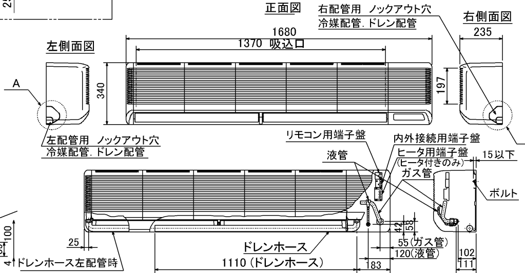
下面図
