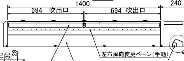
下面図
