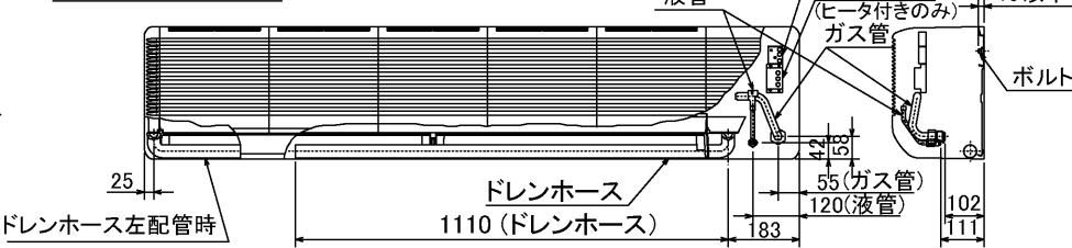
下面図
