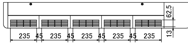
正面図
