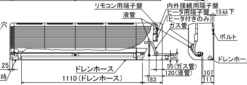
下面図
