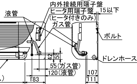
6. 後配管取出口
