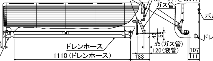
下面図
