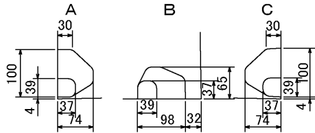
配管用ノックアウト穴詳細図
