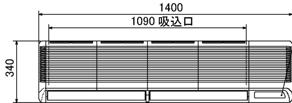
正面図
