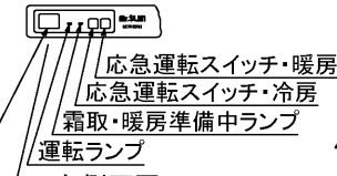
右側面図
