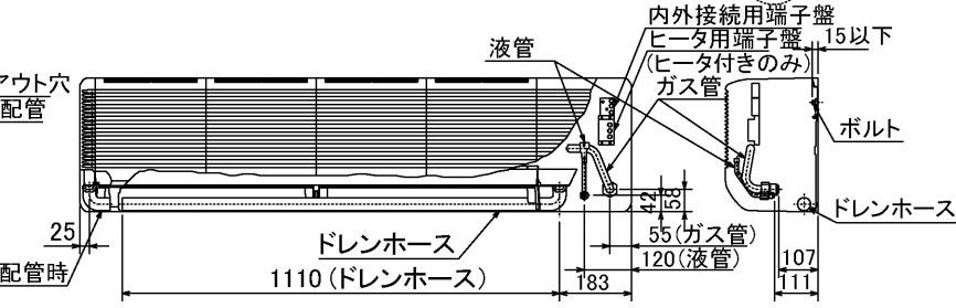
下面図
