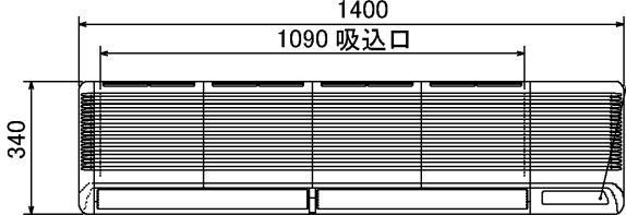
正面図
