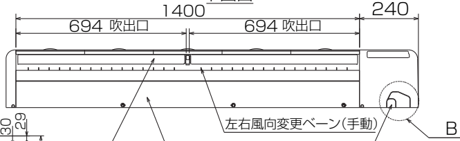
下面図
