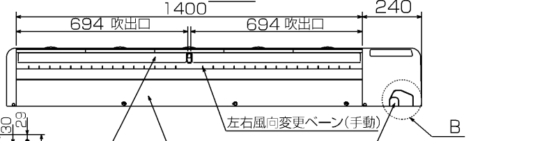
下面図
