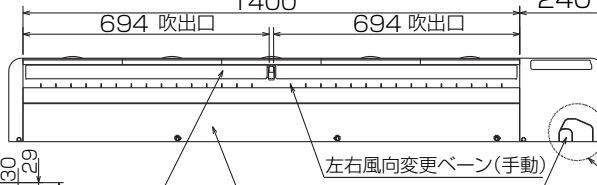
下面図
