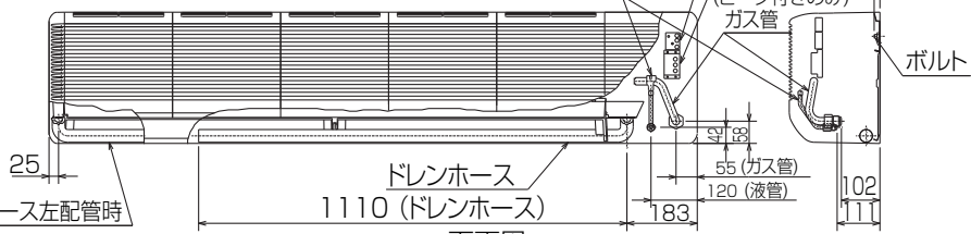
下面図
