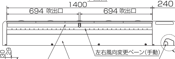
下面パネル (左配管作業時取外し可) オートベーン(上下風向変更ベーン:電動)
