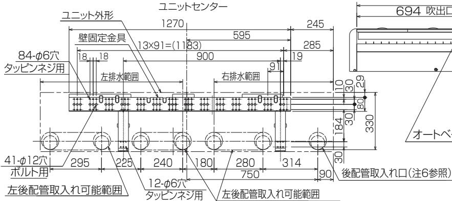
下面パネル (左配管作業時取外し可) オートベーン(上下風向変更ベーン:電動)
