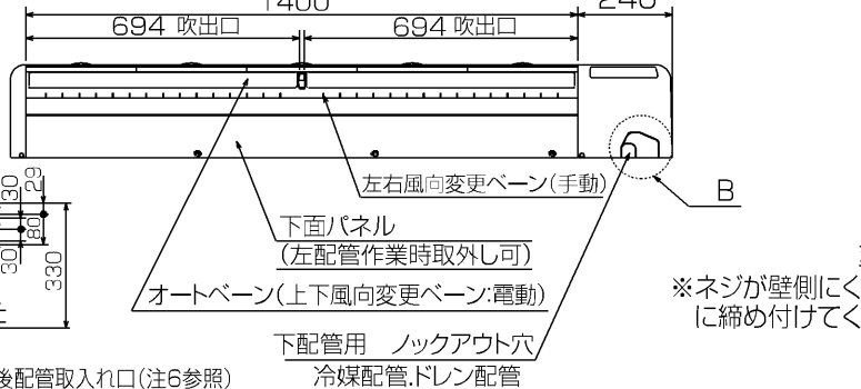
下面図
