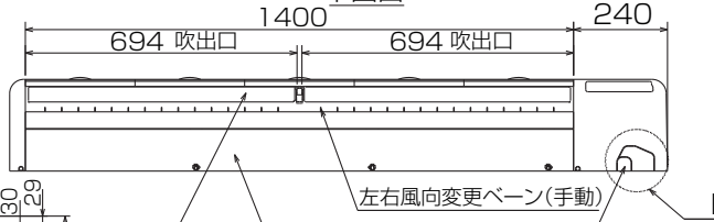
下面図
