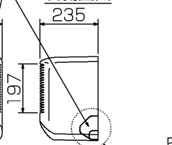
右側面図
