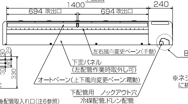
下面図
