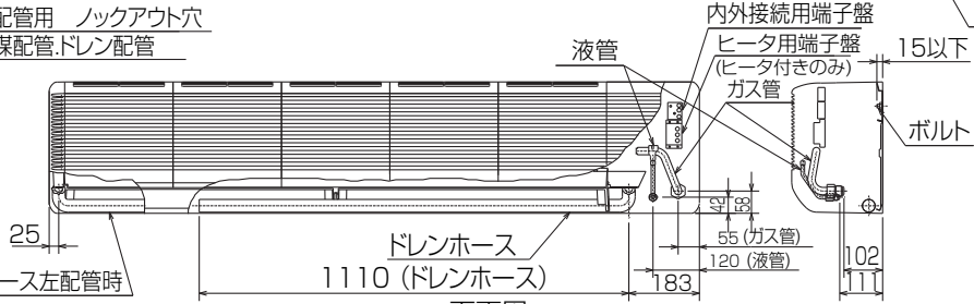
下面図
