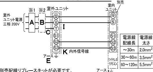
(3) 室 外 ユ ニ ッ ト 以 上 室 内 ユ ニ ッ ト に 電 源 を 供 給 す る 方 式
