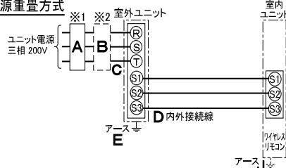
(1) 電 源 重 置 方 式
