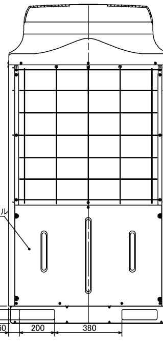
背面図
