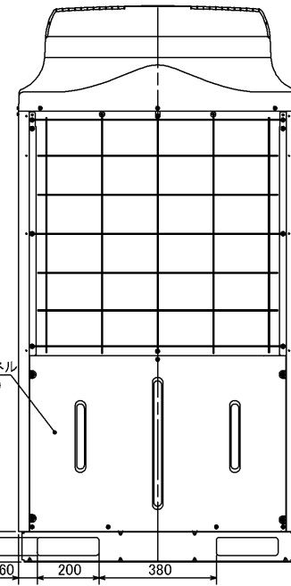
背面図
