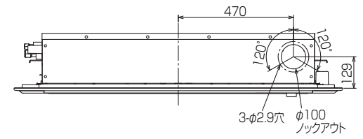
正面図 前吹きダクト接続口詳細図
