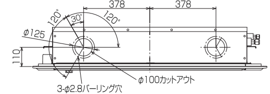
正面図 加湿器(別吊り方式)用ダクト接続口詳細図
