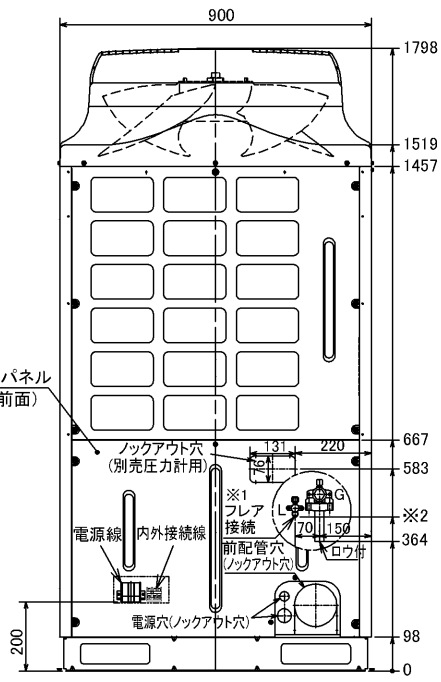
正面図
