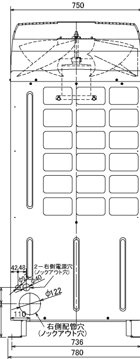
右側面図
