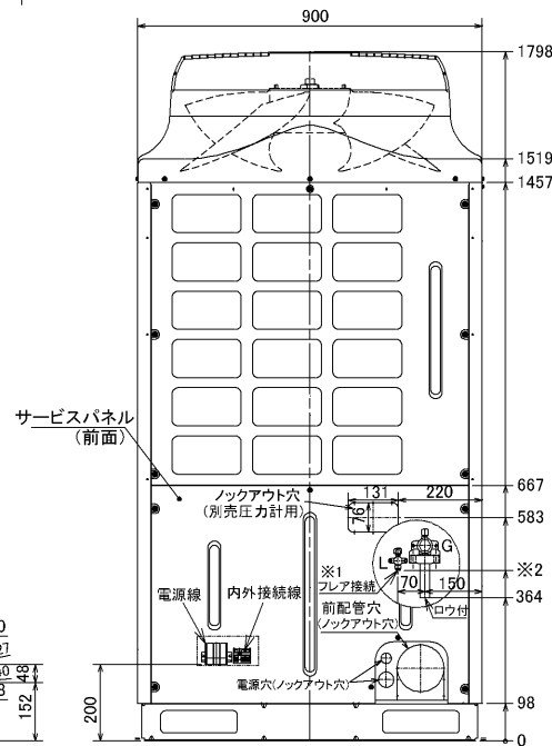
※1 液配管フレア接続 224形: 3/8F...※2 435 280形: 1/2F...※2 419
