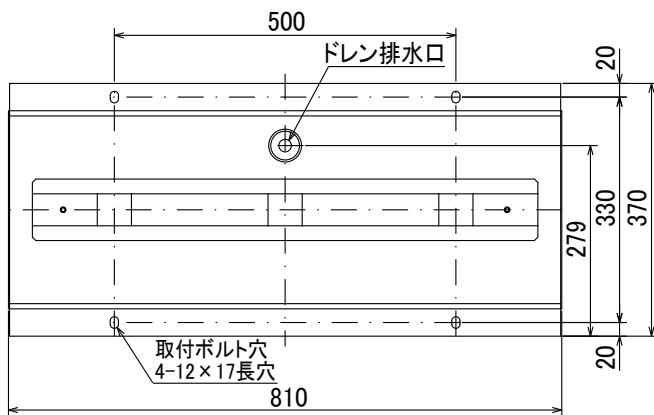
室外ユニット吹出側
