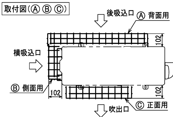
(C)正面用
