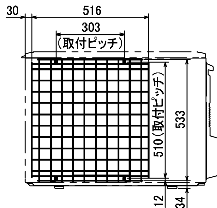
(C)正面用
