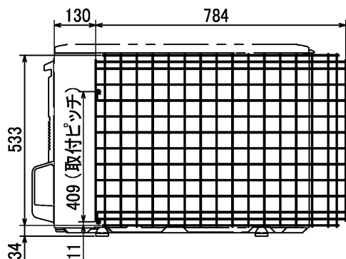
(A)背面用
