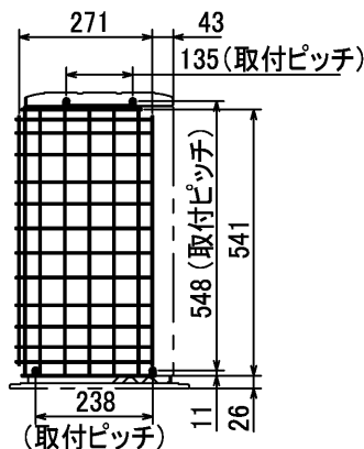
(B)側面用
