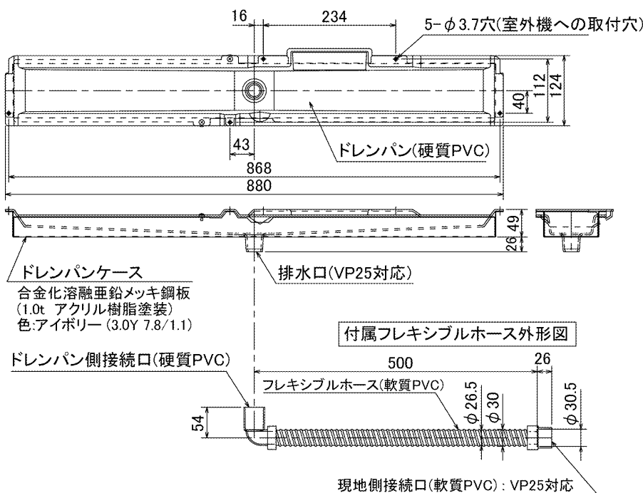
取付状態図
