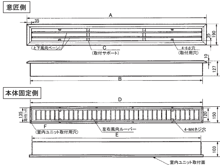
変化寸法表
