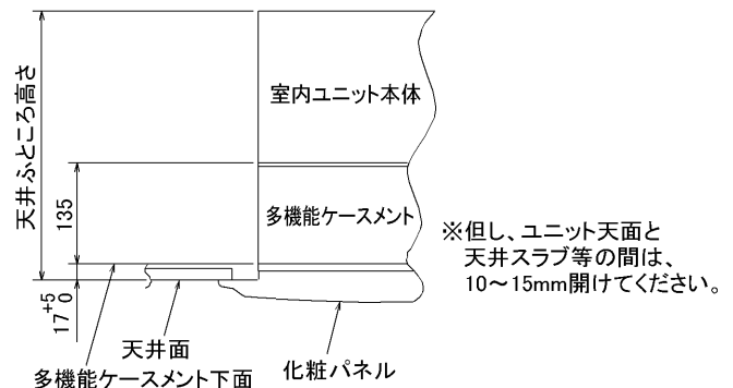
据付状態図
