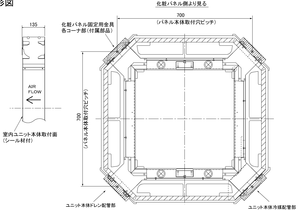
据付状態図
