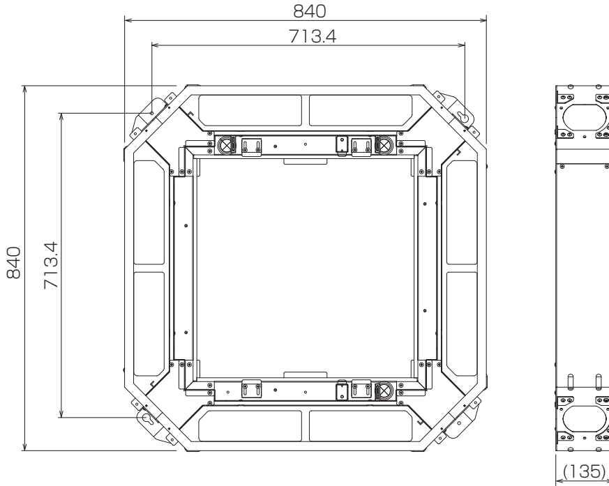
外気取入口詳細図(4箇所)
