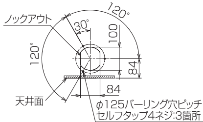
外気取入口詳細図(4箇所)
