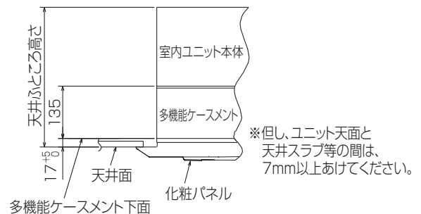
据付状態図
