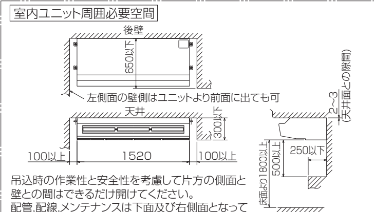
室内ユニット周囲必要空間 R01N812-2
