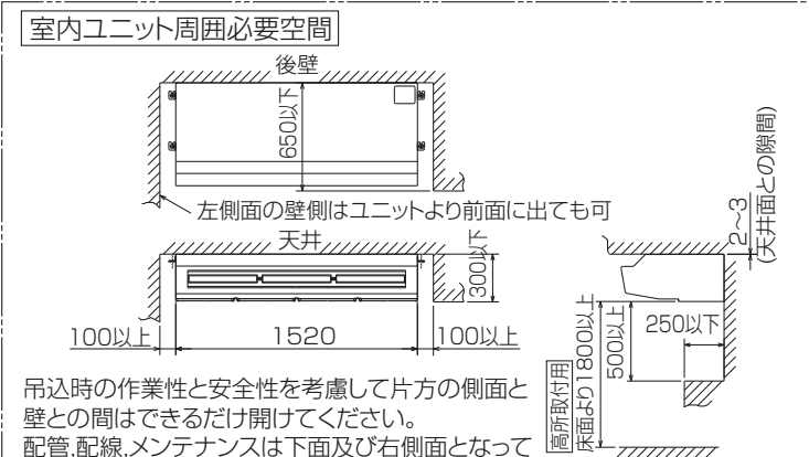
室内ユニット周囲必要空間 吊込時の作業性と安全性を考慮して片方の側面と壁との間はできるだけ開けてください。 配管、配線、メンテナンスは下面及び右側面となっておりますので上記スペースを確保してください。 RG01N812-2
