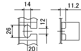
A(吊りボルト用穴詳細図)
