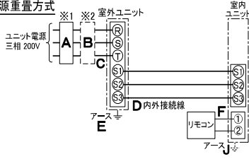
(1)電源重畳方式
