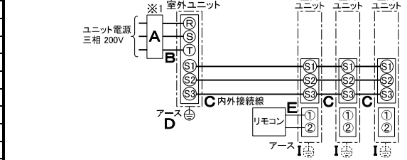
(1)電源重畳方式
