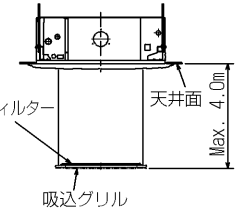
カンタン自動パネル 吸込グリル昇降寸法
