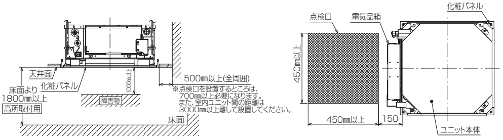
詳細図(1:2)
