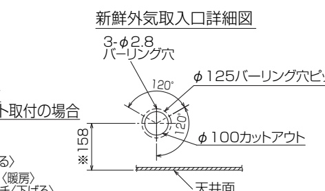
新鮮外気取入口詳細図
